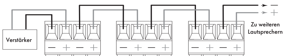
Paralleles Schaltschema
